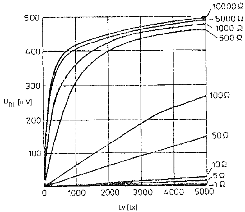
Spadek napięcia na rezystancji obciążenia w zależności od intensywności promieniowania świetlnego
